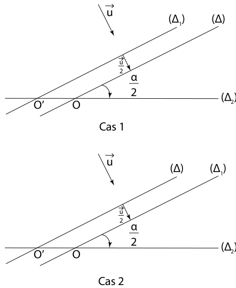
FIGURE 7 – Composée d’une rotation et d’une réflexion
