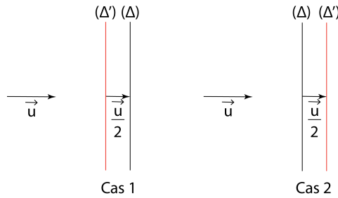
FIGURE 5 – Composée d'une translation et d'une réflexion
